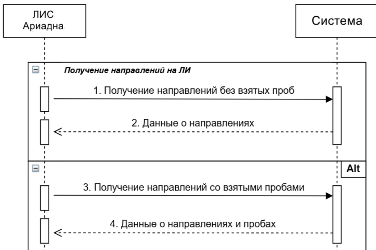
Рисунок 4 – Диаграмма взаимодействия при выполнении сценария "Получение данных о направлениях на лабораторные исследования"
